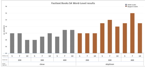
(d) Fasttext models SA results For Books corpus
