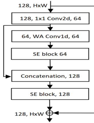
(d) Proposed block.
