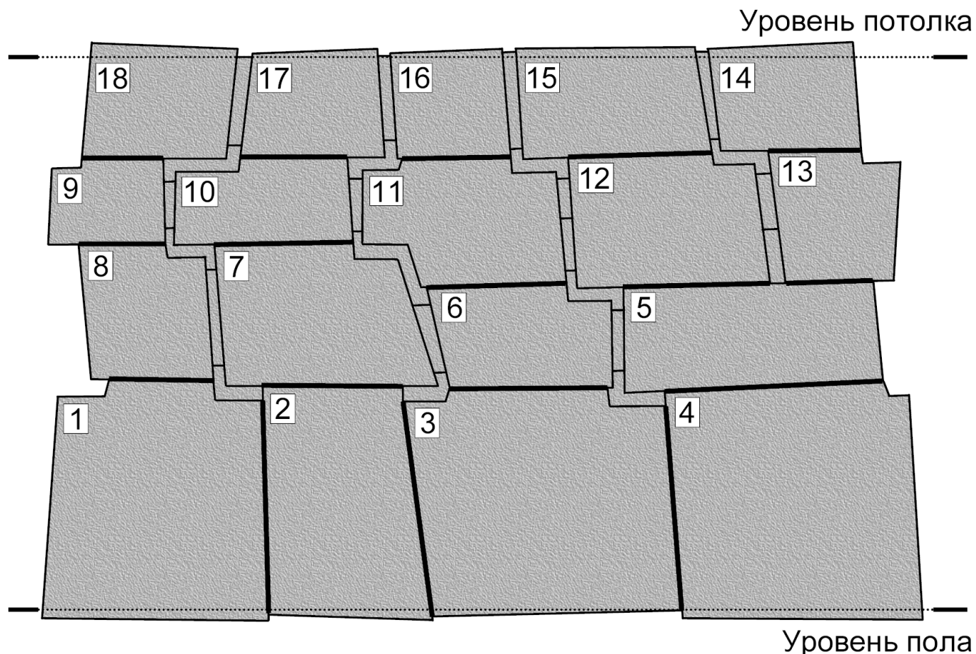
Рис. 1. Вероятный вид полученной литьем полигональной кладки из плотно примыкающих друг к другу блоков. Небольшие блоки, отливаемые на завершающем этапе, предназначены для выборки межблочных зазоров, возникающих из-за усадки бетона в больших блоках. Участки примыкания между большими блоками (показаны жирной линией) лишь изображены прямолинейными с нулевыми зазорами, в реальности из-за неравномерной усадки эти участки, строго говоря, являются криволинейными и примыкания всегда имеют непостоянный зазор. Зазоры тем больше, чем больше коэффициент усадки и размеры блока. Отклонения блоков от границ уровней пола и потолка вследствие усадки преувеличены для большей наглядности. Недостатком кладки является довольно слабая перевязка блоков. Цифрами показан порядок установки больших блоков.
