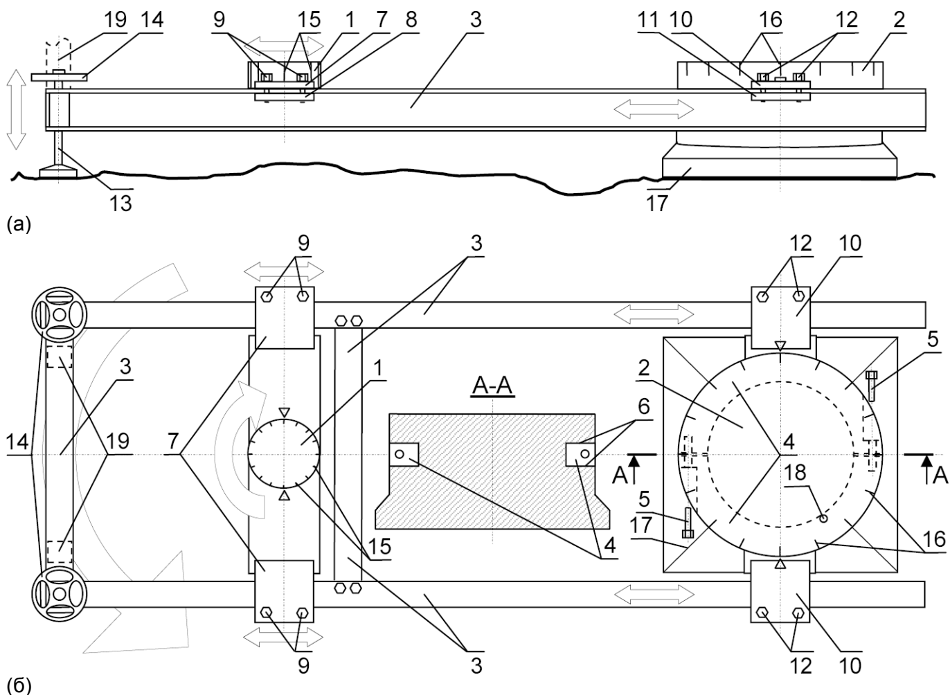
Рис. 4. Планетарный строительный 3D-пантограф: 1 – поворотная платформа, на которую устанавливается уменьшенная глиняная модель каменного блока; 2 – неподвижное основание, на которое устанавливается обрабатываемый каменный блок; 3 – рама пантографа, собранная из двутавровых балок; 4 – разъемный подшипник скольжения, состоящий из двух половин кольца, обеспечивающий возможность поворота пантографа вокруг неподвижного основания 2 в горизонтальной плоскости; 5 – болты, соединяющие две половины кольца разъемного подшипника скольжения 4; 6 – кольцевая канавка прямоугольного сечения в цилиндрической части неподвижного основания 2, в которую вставляется кольцо разъемного подшипника скольжения 4; 7 – плоские пластины, посредством которых поворотная платформа 1 крепится к раме 3 с помощью струбцин 8 и болтов 9; 10 – плоские пластины, посредством которых кольцо разъемного подшипника скольжения 4 крепится к раме 3 с помощью струбцин 11 и болтов 12; 13 – винтовые опоры для выравнивания поворотной платформы 1 в горизонтальной плоскости; 14 – рукоятки винтовых опор; 15 – риски 11.25°-секторов, на которые разделён круг поворотной платформы 1; 16 – риски 11.25°-секторов, на которые разделён круг неподвижного основания 2; 17 – широкая опорная часть неподвижного основания 2; 18 – отверстие с пробкой для смазки разъемного подшипника скольжения; 19 – места установки вертикальной рамы, на которой закреплена стрела пантографа с параллелограммным механизмом и противовес (см. Рис. 2). Вид пантографа (а) спереди, (б) сверху.
