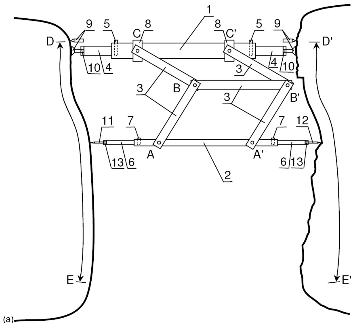
Рис. 5. Транслятор рельефа: 1 – несущий стержень; 2 – измерительный стержень; 3 – двойной параллелограммный механизм ( AB=A'B'=BC=B'C' , AA'=BB'=CC' ); 4 – выдвижные секции для грубой установки длины несущего стержня; 5 – штифты, фиксирующие положения выдвижных секций несущего стержня; 6 – выдвижные секции для грубой установки длины измерительного стержня; 7 – штифты, фиксирующие положения выдвижных секций измерительного стержня; 8 – цилиндрические шарниры, обеспечивающие свободное вращение измерительного стержня вместе с двойным параллелограммным механизмом вокруг несущего стержня; 9 – опоры (с заострением или с плоской подошвой) несущего стержня, вывинчивая которые несущий стержень крепится в распор между двумя сопрягаемыми каменными блоками; 10 – контргайки, фиксирующие положения опор несущего стержня; 11 – щуп измерительного стержня; 12 – указатель измерительного стержня; 13 – контргайки, фиксирующие положение щупа и указателя измерительного стержня; 14 – цилиндрические шарниры, обеспечивающие свободное вращение измерительного стержня вокруг своей оси; DE – произвольно-обработанный участок боковой поверхности предыдущего каменного блока; D'E' – обрабатываемый с использованием транслятора участок боковой поверхности текущего каменного блока. Установка несущего стержня в распор между блоками (а) перпендикулярно сопрягаемым поверхностям на опоры с плоской подошвой, (б) под углом к сопрягаемым поверхностям на опоры с заострениями. (б) Транслятор с дополнительными шарнирами 14, изогнутым щупом 11 и изогнутым указателем 12 для работы с U-образными выемками.
