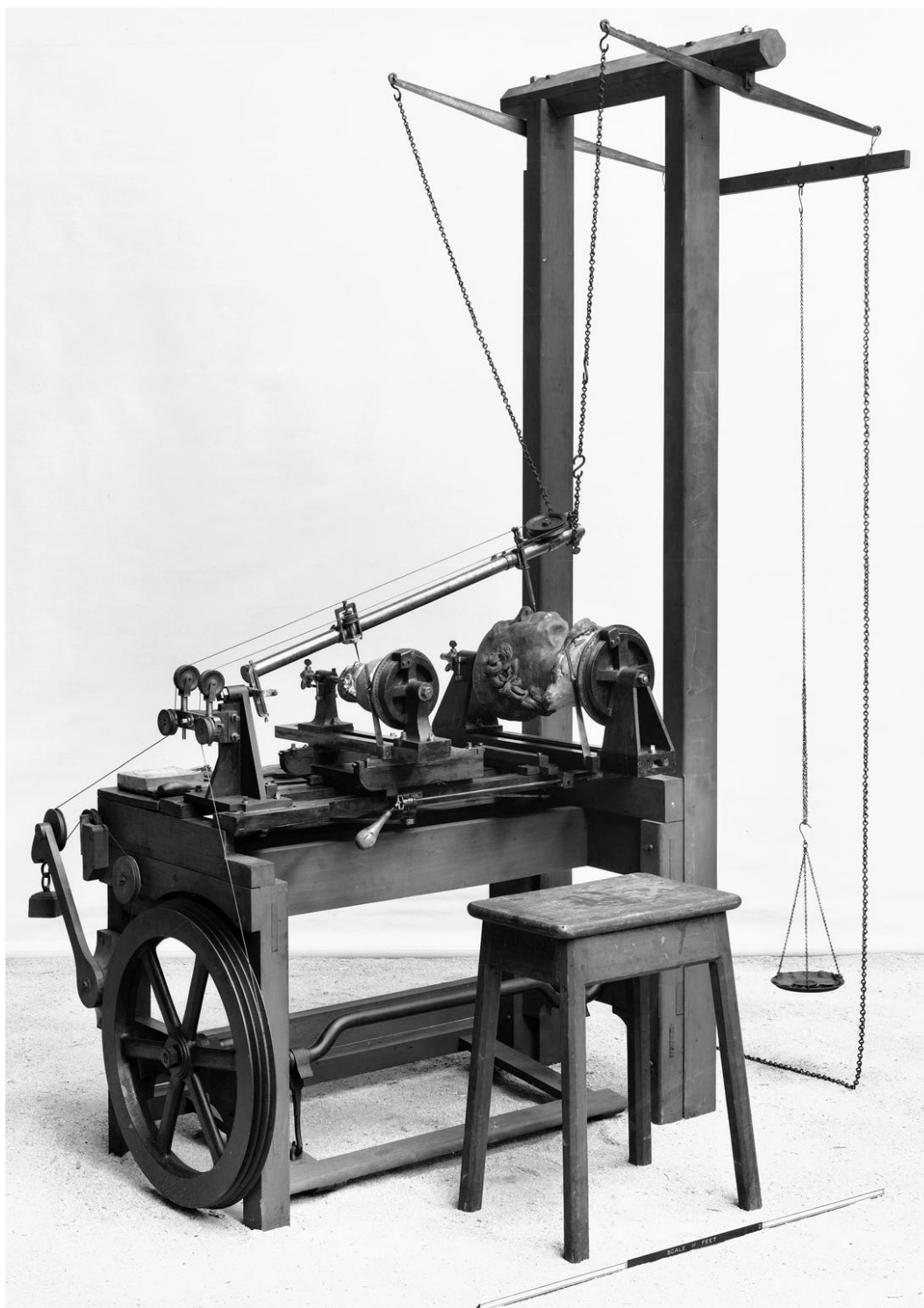
Фото. 21. 3D-пантограф, разработанный и построенный Д. Уаттом, 1807 г. Механизм предназначался для автоматического изготовления уменьшенных копий скульптур (Музей Науки, Лондон, sciencemuseumgroup.org.uk ).
