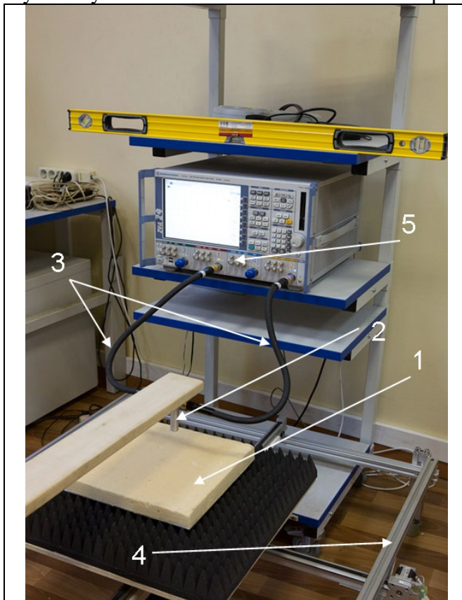
Fig. 23 Experimental high precision HSR system; 1) test sample, 2) antenna, 3) cables, 4) electromechanical scanning bed, 5) VNA (ZVA 24).
