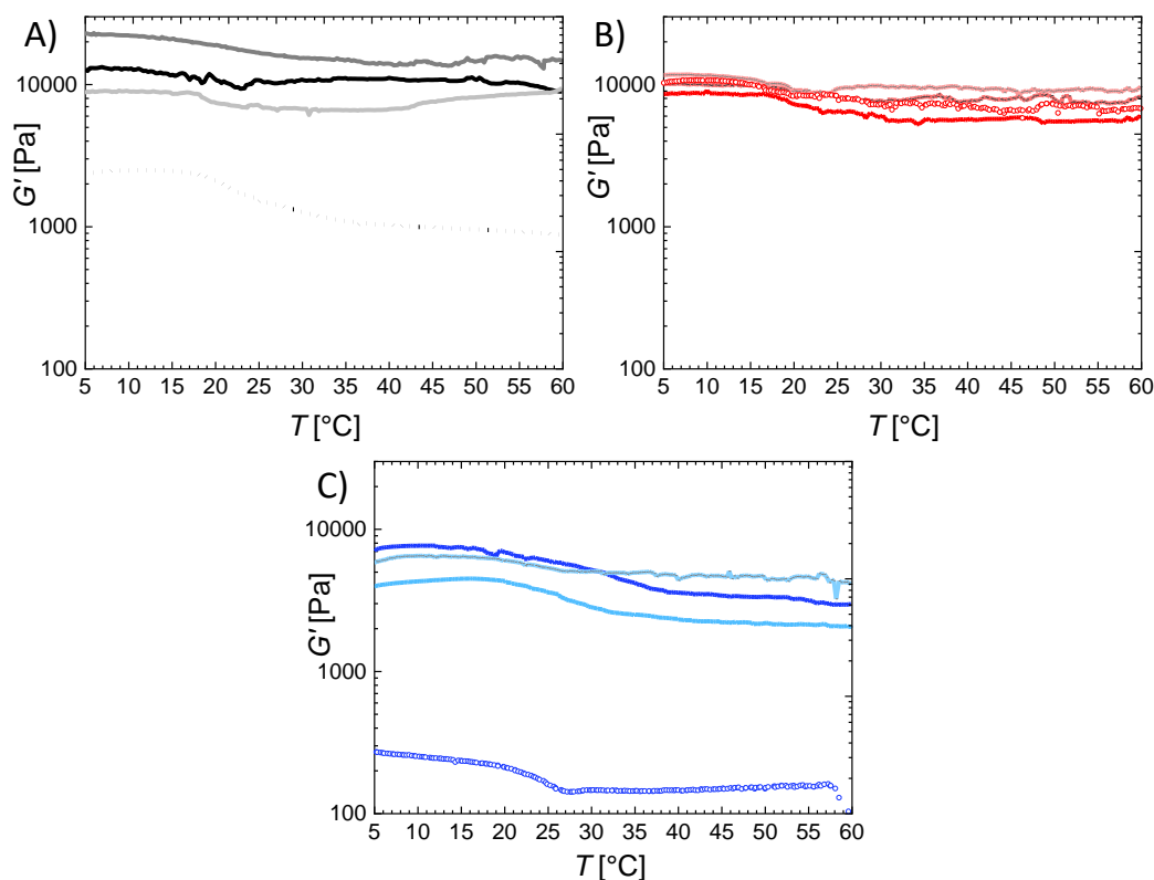
Figure 3. Storage modulus G' of (A) G20_OEG1000( z ), (B) G20_OEG1500( z ) and (C) G20_OEG3400( z ) hydrogels at different temperatures. z = 0.75 (---), 1 (---), 2 (---), and 3 (-○-○-○).
