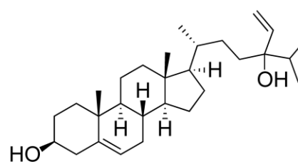
Saringosterol
