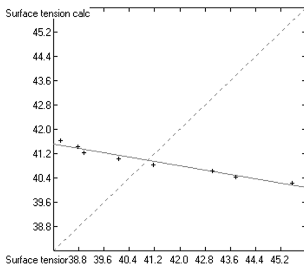
Fig. 4e: n-Alkyl \alpha,o -dinitrate
