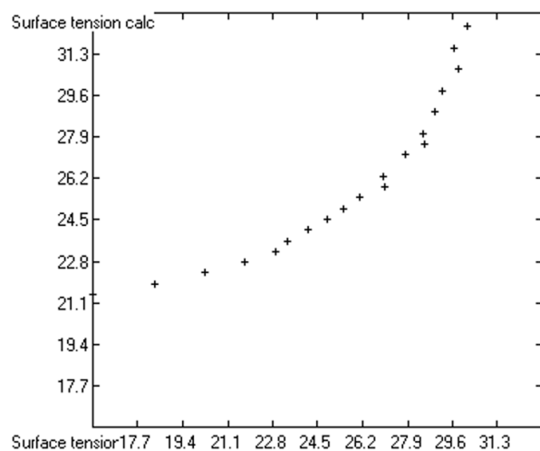
Fig. 4c: n-Alkanes
