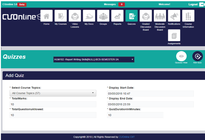
Fig. 8: Quizzes Tab
