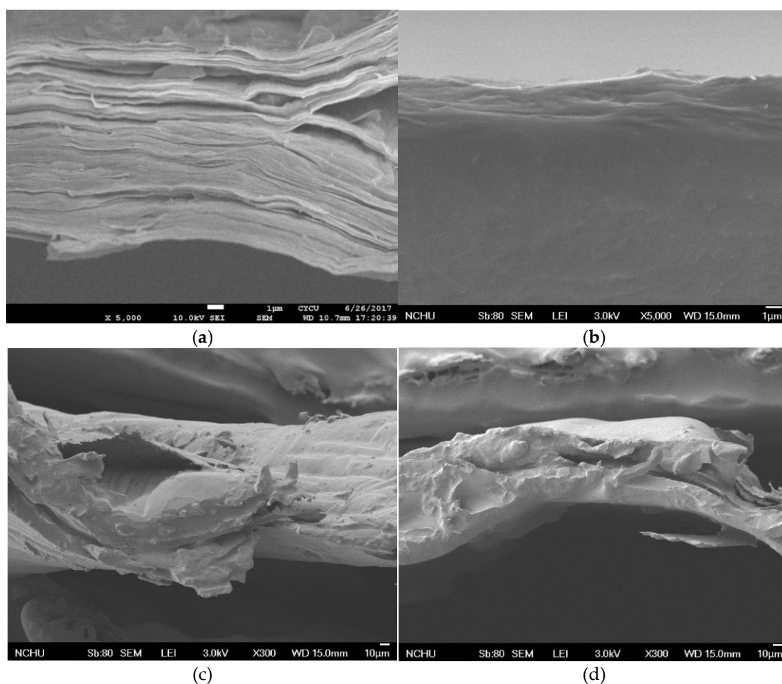
Figure 4. Micrographs of diaphragms (a) GOP-T3-WF3, (b) GOPC-T3-WF3, (c) GOPC-C-T3-WF3 and (d) GOPC-L-T3-WF3.
