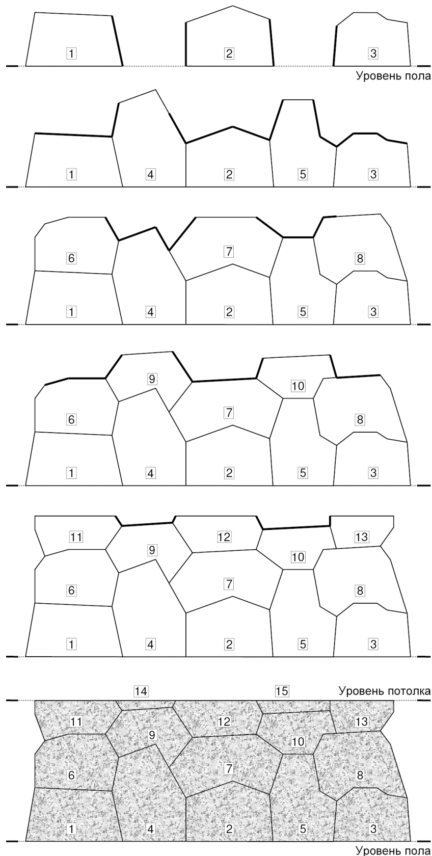
Рис. 3. Способ укладки полигональных блоков, сочетающий элементы способов реплики, глиняной модели и 3D-пантографа. Участки, по которым выполняется сопряжение каменных блоков, показаны жирной линией. Цифры обозначают порядок установки блоков.
